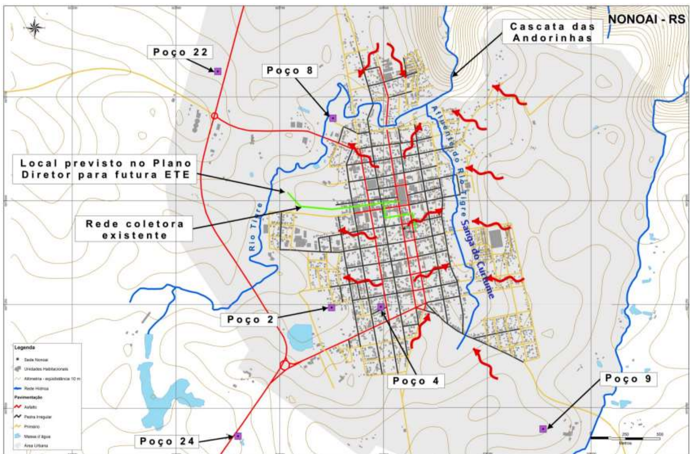
Figura 47: Localização dos poços, da rede coletora de esgoto sanitário e indicação do sentido de escoamento das águas pluviais.
